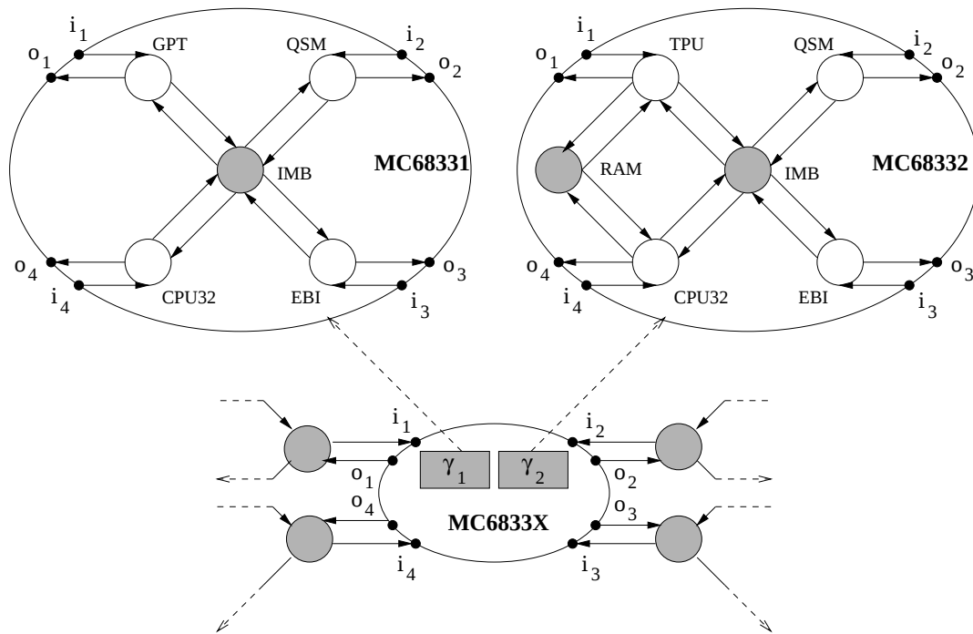
Abbildung 3: Entwurfsalternativen einer funktionalen Ressource (Mikrocontroller)
